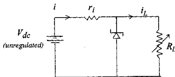
Fig. A Zener voltage regulator
